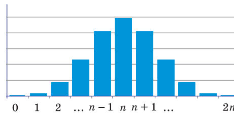
Рис. 2. Распределение Y
