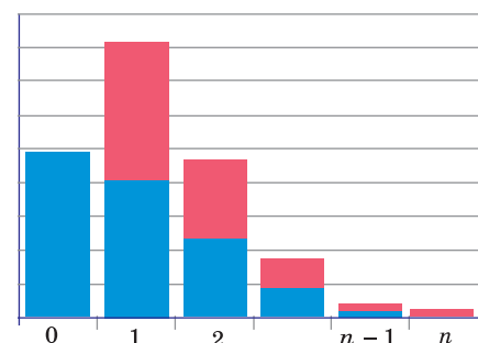
Рис. 3. Распределение X
